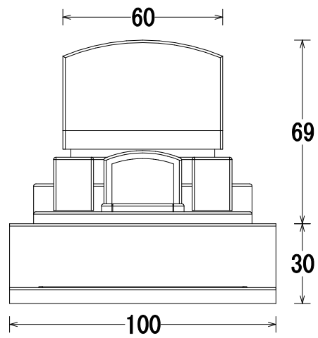
正面図
