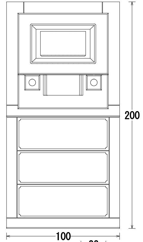
平面図
